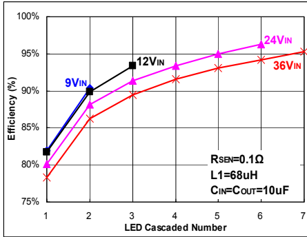
Fig 16. I_{OUT}=1A
