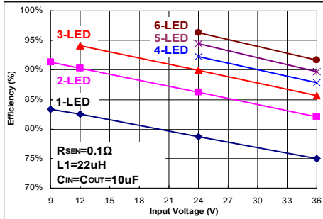
Fig 4. I_{OUT}=1A
