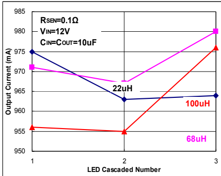
Fig 49. I_{OUT}=1A
