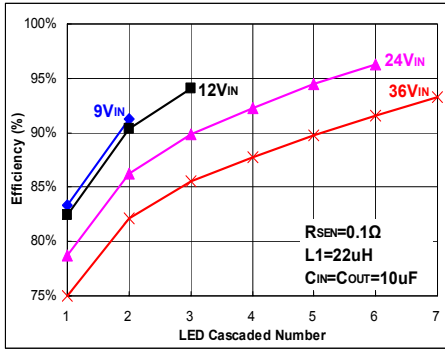
Fig 13. I_{OUT}=1A
