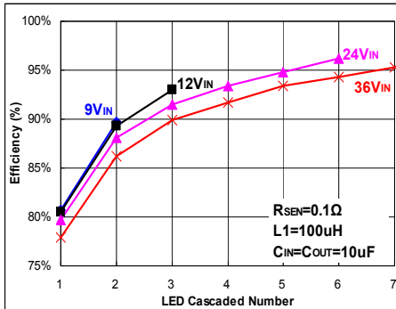
Fig 19. I_{OUT}=1A
